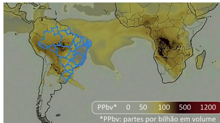
Concentração de CO 2 por queimadas entre África e Brasil em 30 de agosto de 2019
