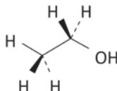
Etanol
