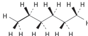
n-hexano
